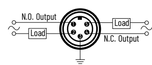
Figure 53. Mini QD Style – N.O. or N.C.
