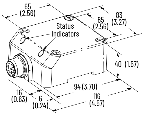
Figure 119. Mini QD Style
