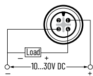
Figure 57. Pico QD Style – N.O.
