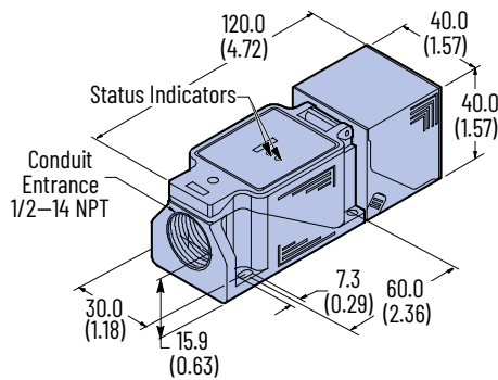
Figure 140. Conduit Style
