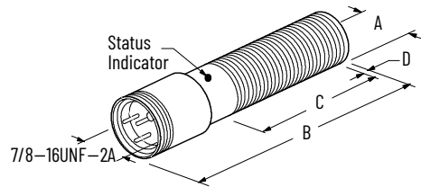
Figure 109. Mini QD Style
