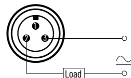
Figure 76. Mini QD Style – N.O.
