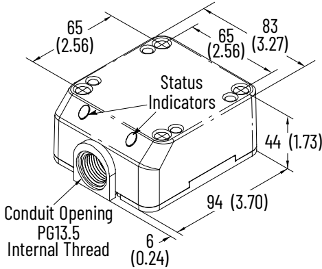
Figure 127. Conduit Style PG13.5
