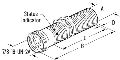
Figure 79. Mini QD Style
