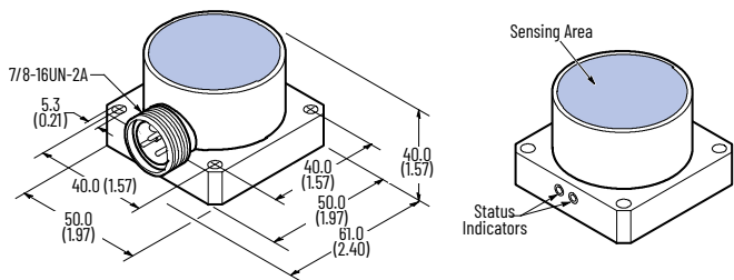
Figure 132. Mini QD Style
