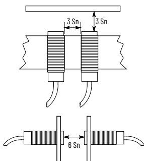
Figure 24. Tubular Style Extended Sensing (Bul. 872C)
