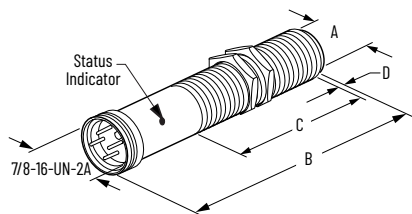
Figure 49. Mini QD Style
