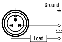
Figure 86. Mini QD Style – N.O.
