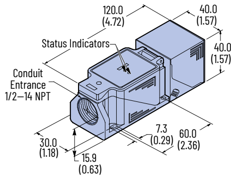
Figure 138. Mini QD Style
