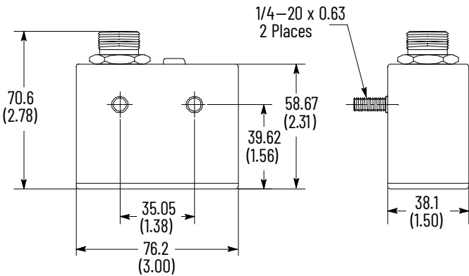
Figure 143. Long -Range Mini QD Style
