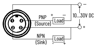
Figure 152. Mini and M12 Micro QD Style
