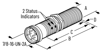
Figure 51. Mini QD Style
