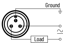
Figure 68. Mini QD Style – N.O. or N.C.
