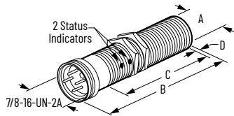
Figure 84. Mini QD Style
