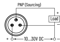
Figure 57. Pico QD Style – N.O.
