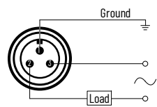
Figure 144. Long -Range Mini QD Style
