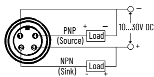
Figure 148. Mini QD Style
