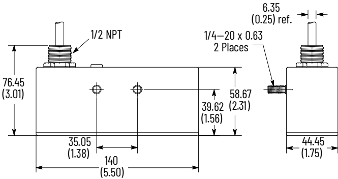
Figure 146. Mini QD Style
