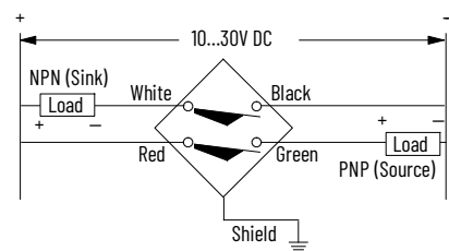
Figure 148. Mini QD Style
