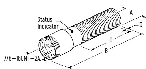
Figure 106. Mini QD Style
