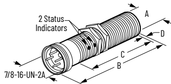
Figure 65. Mini QD Style
