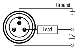
Figure 166. Mini QD Style – Normally Open
