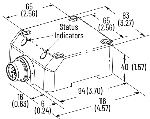
Figure 128. Mini QD Style
