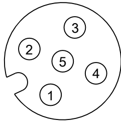
Fig. 28: M12 socket
