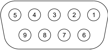
Fig. 15: D-sub socket, 9-pin
