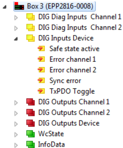
Fig. 3: EPP2816-0008, DIG Inputs Device
